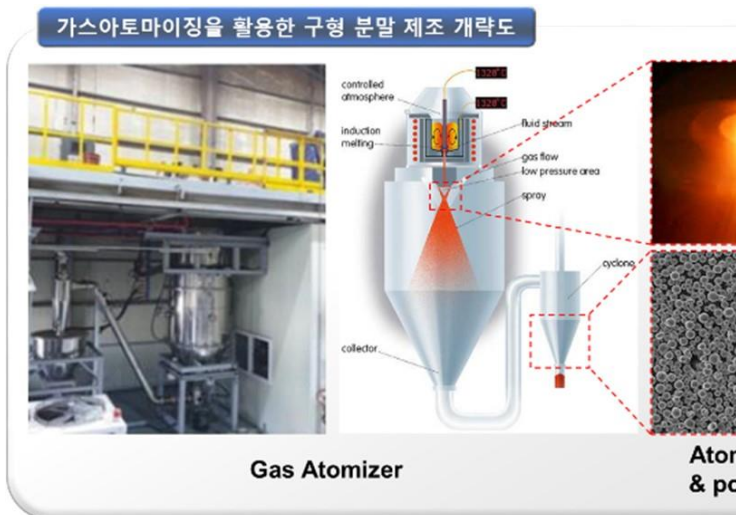
분말 합금 관련 제조 개략도
